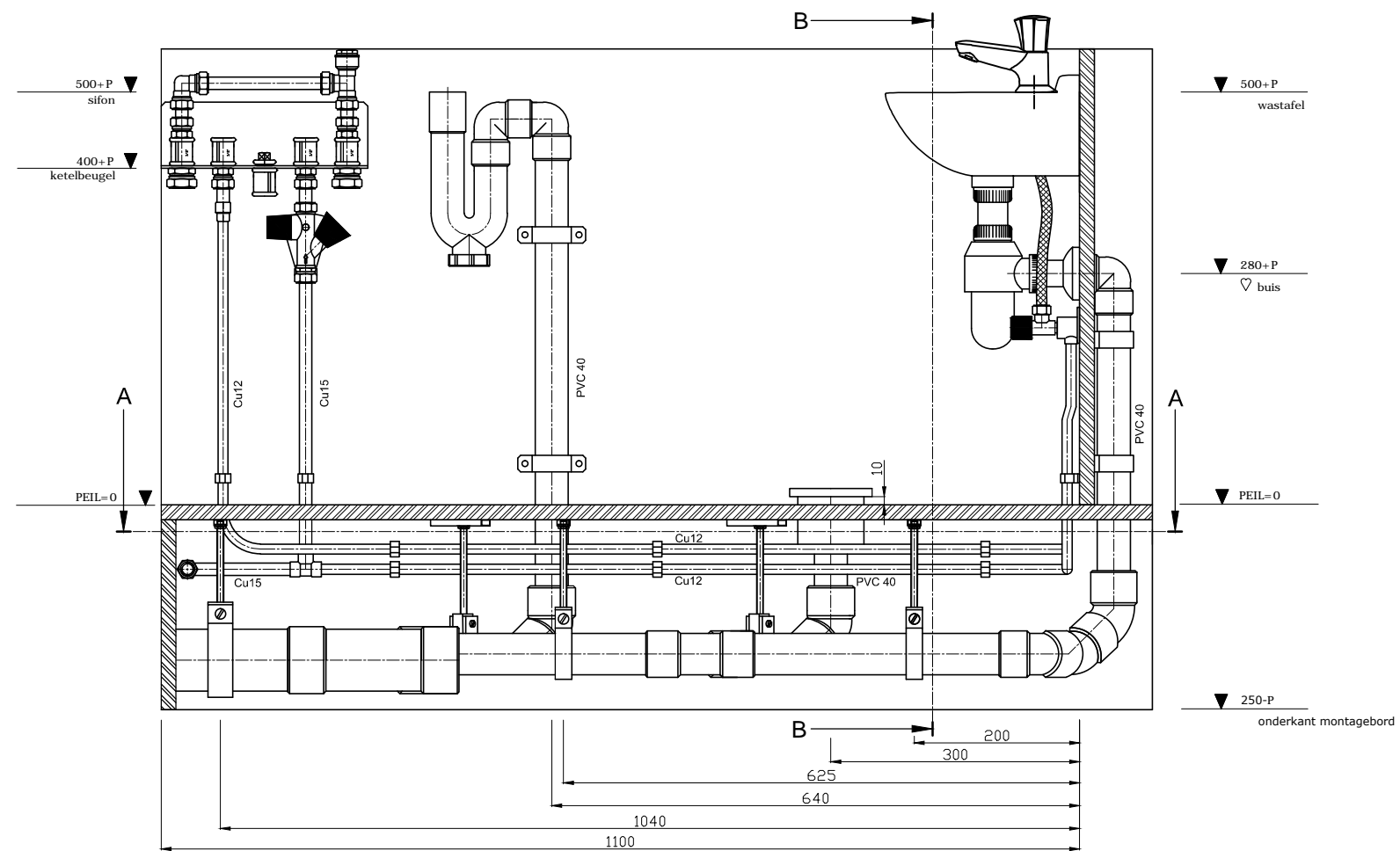
vooraanzicht
